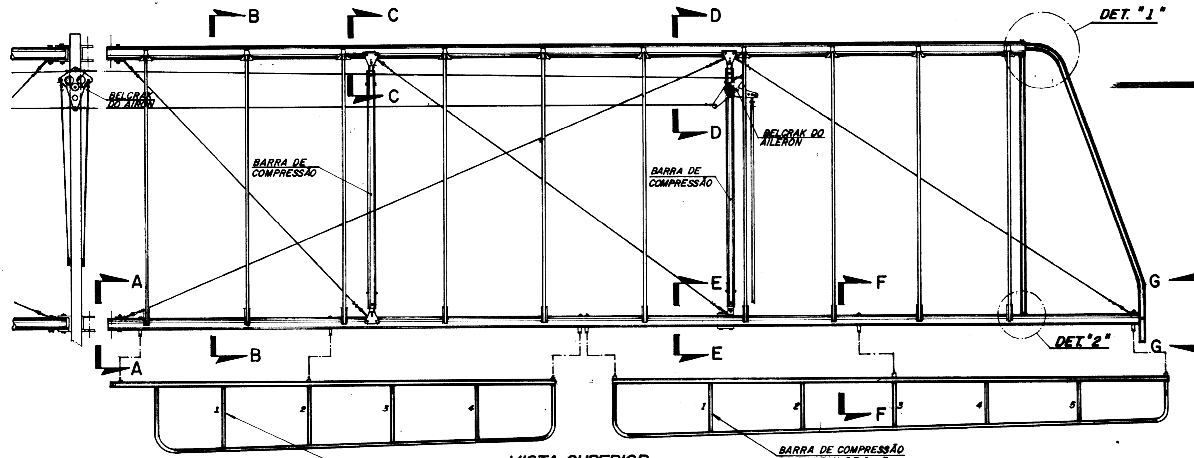
VISTA SUPERIOR ASA DIREITA
