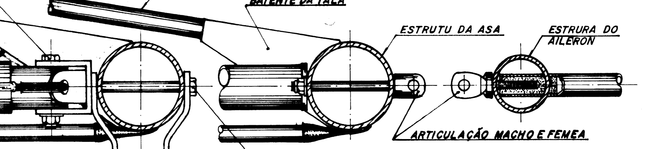
CORTE F-F
