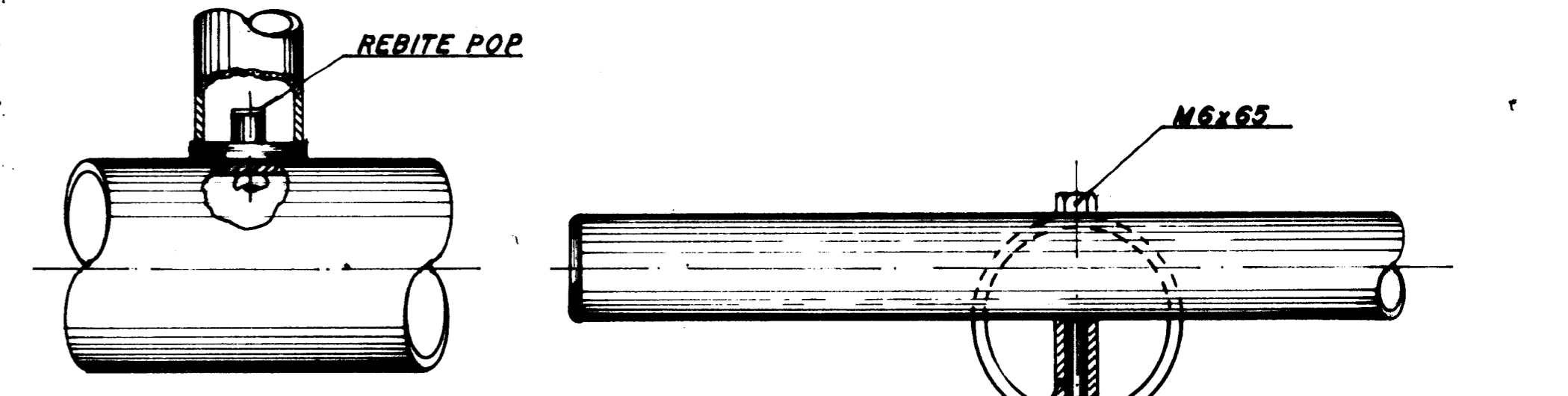
DETALHE "2"
